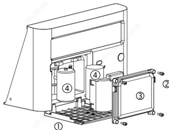
Рисунок 5. Замена элемента питания счетчика исполнения И1, И3
