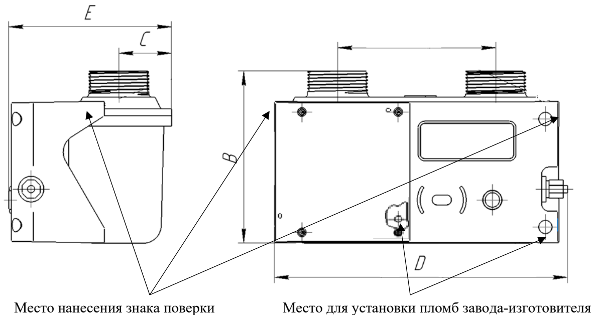
Рисунок 1. Счетчик ВК-У G1,6; G2,5; G4; G6 «К» исполнение И1
