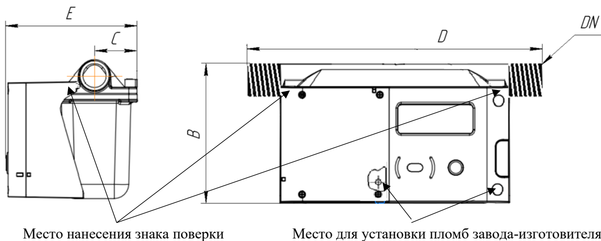
Рисунок 3. Счетчик ВК-У исполнение И3
