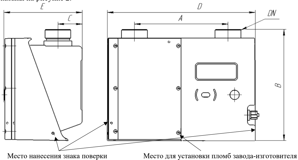
Рисунок 2. Счетчик ВК-У G6 «Б»; G10 исполнение И1
