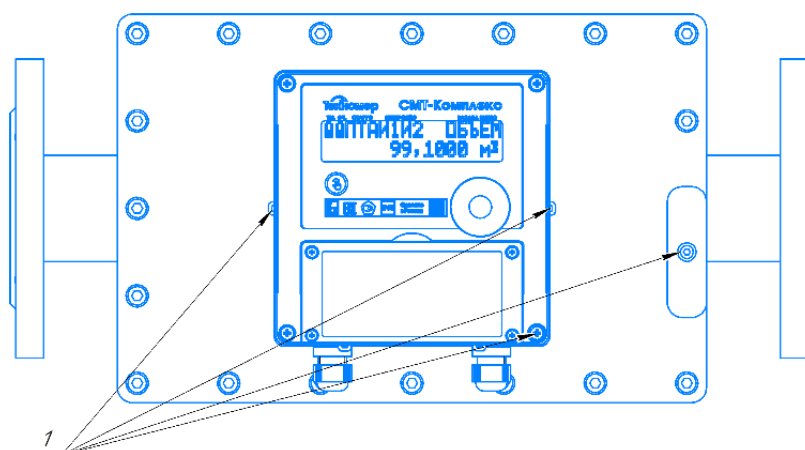
Рисунок 15.2 – Схема пломбировки СМТ-Комплекс G40, G40-2, G65, G100 1 – места установки пломбы поверителя, 2 – места установки пломбы поставщика газа
