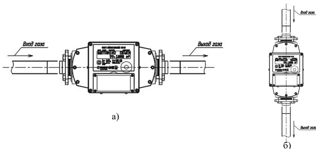
Рисунок Б3 – пример монтажа СМТ-Комплекс в отапливаемых помещениях.
