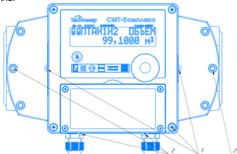
Рисунок 15.1 – Схема пломбировки СМТ-Комплекс G4-G25
