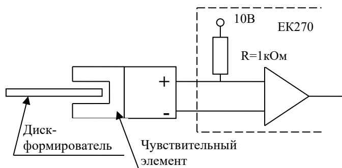
Рисунок 20. Схема среднечастотного датчика импульсов R300
