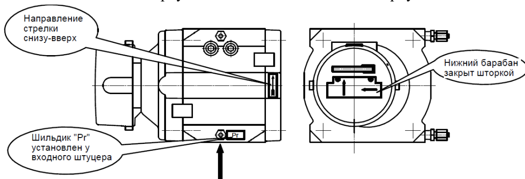
Рисунок 7. Установка шторки и шильдиков при направлении потока газа снизу-вверх. Счетный механизм повернут на 90°
