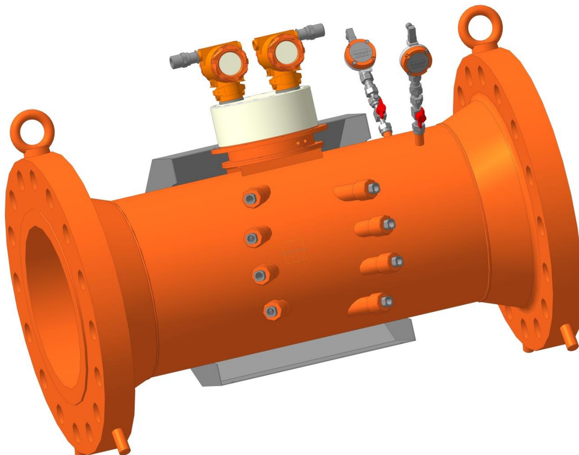
Рисунок Б.11 - Расходомер - счетчик газа ультразвуковой исполнение с дублированием dB
