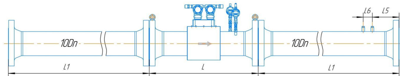
Рисунок Д.25 – Монтаж реверсивного расходомера класса точности В/В* (1,0/1,2*% - 1,0/1,2*%) для исполнения с дублированием с типом присоединительных фланцев по ГОСТ 33259
