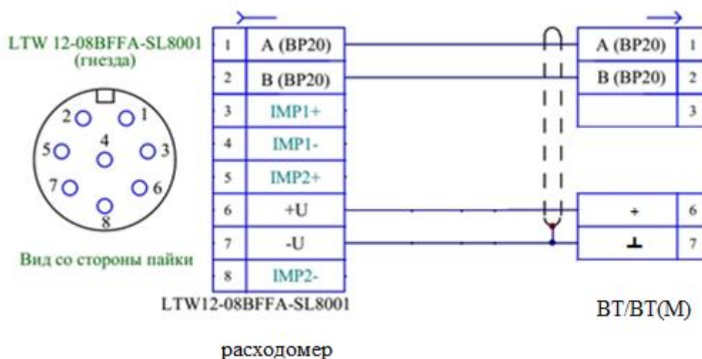
Рисунок Г.6 – Кабельный разъем для подключения ПТ (ХS1) в зависимости от исполнения корпуса
