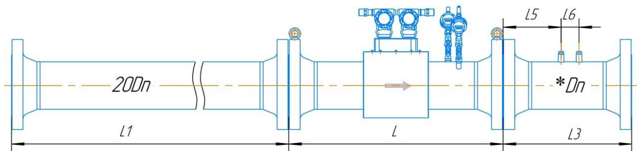
Рисунок Д.26 – Монтаж расходомера классов точности А/А* (0,5/0,7% - 0,3/0,5%) и Б/Б (0,5/0,7% - 0,5/0,7%) для исполнения с дублированием по стандарту ASME B16.5-2003
