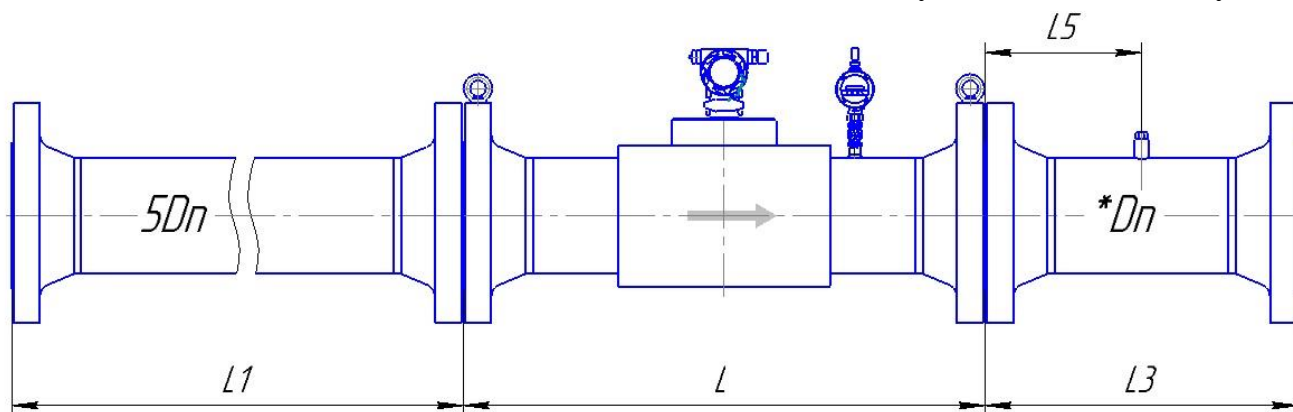
Рисунок Д.6 – Монтаж расходомера класса точности Г/Г* (2,0/2,2*% - 1,0/1,2*%)
