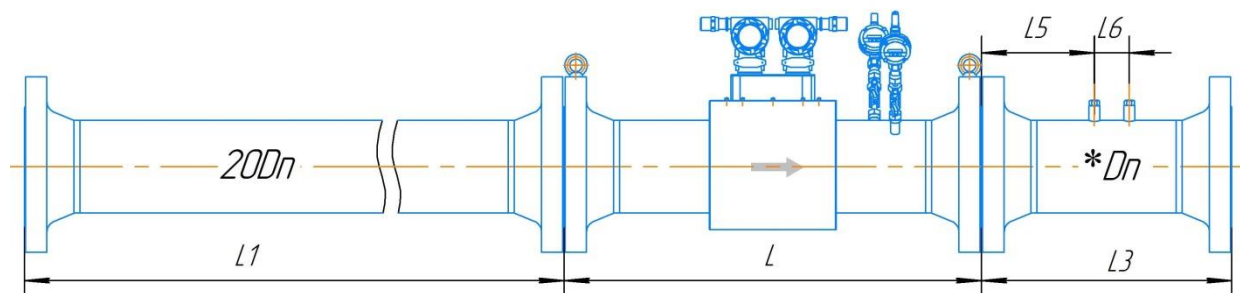
Рисунок Д.19 – Монтаж расходомера классов точности А/А* (0,5/0,7% - 0,3/0,5%) и Б/Б (0,5/0,7% - 0,5/0,7%) для исполнения с дублированием с типом присоединительных фланцев по ГОСТ 33259
