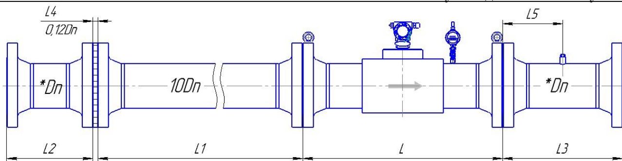
Рисунок Д.2–Монтаж расходомера со струевыпрямителем со вставкой 2Dn классов точности А/А*(0,5/0,7*% - 0,3/0,5*%) и Б/Б (0,5/0,7*%- 0,5/0,7*%) для исполнения корпуса V и С с типом присоединительных фланцев по ГОСТ 33259
