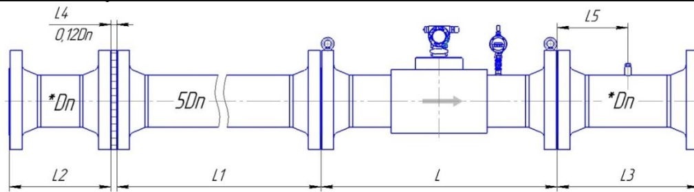
Рисунок Д.6.1 – Монтаж расходомера со струевыпрямителем со вставкой 2Dn рекомендуемая схема минимальных длин прямолинейных участков измерительного трубопровода (ПУИТ) для монтажа расходомера класса точности Г/Г*(2,0/2,2*% - 1,0/1,2*%) для исполнения корпуса V и С с типом присоединительных фланцев по ГОСТ 33259
