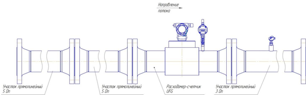
Рисунок 2.15 – Пример составного прямолинейного участка длиной 10Dn
