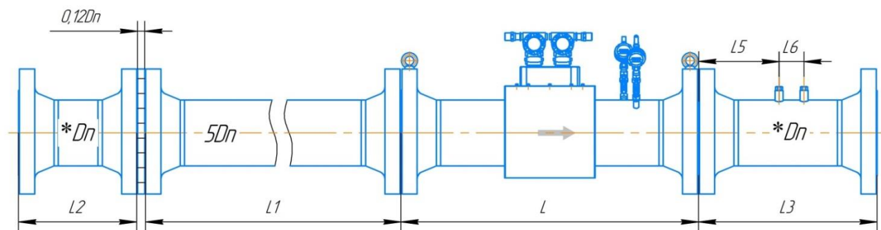
Рисунок Д.30 – Монтаж расходомера со струевыпрямителем со вставкой 2Dn класса точности В/В* (1,0/1,2% - 1,0/1,2%) для исполнения с дублированием по стандарту ASME B16.5-2003 (* погрешность в зависимости от метода проведения поверки – проливной / имитационный (первичный имитационный и/или периодический имитационный при условии первичной поверки проливным методом))
