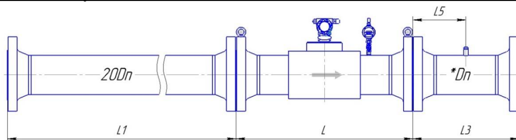
Рисунок Д.10 – Монтаж расходомера классов точности А/А* (0,5/0,7% - 0,3/0,5%) и Б/Б (0,5/0,7% - 0,5/0,7%) для исполнения корпуса V с типом присоединительных фланцев по стандарту ASME B16.5-2003
