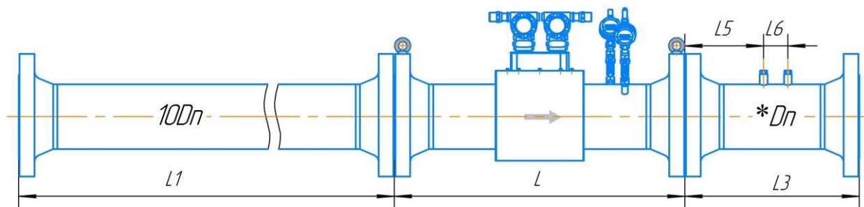
Рисунок Д.29 – Монтаж расходомера класса точности В/В* (1,0/1,2*% - 1,0/1,2*%) для исполнения с дублированием по стандарту ASME B16.5-2003
