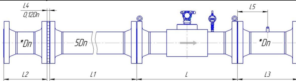
Рисунок Д.14 – Монтаж расходомера со струевыпрямителем со вставкой 2Dn класса точности В/В* (1,0/1,2*% - 1,0/1,2*%) для исполнения корпуса V по стандарту ASME B16.5-2003 (* погрешность в зависимости от метода проведения поверки – проливной / имитационный (первичный имитационный и/или периодический имитационный при условии первичной поверки проливным методом))
