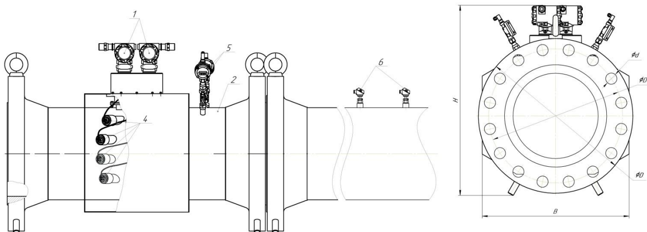
Рисунок Б.11 - Расходомер - счетчик газа ультразвуковой исполнение с дублированием dB
