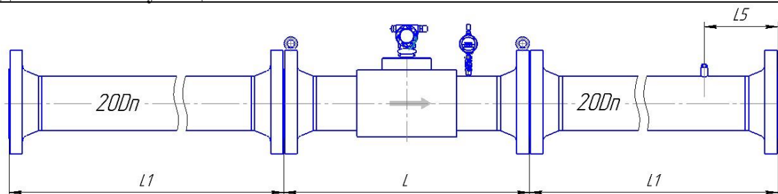
Рисунок Д.16 – Монтаж реверсивного расходомера классов точности А/А* (0,5/0,7% - 0,3/0,5%) и
